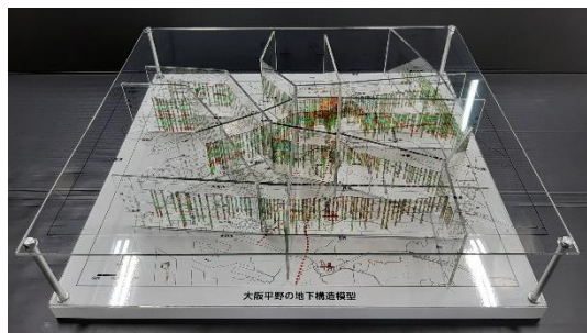
大阪平野の地下構造模型
